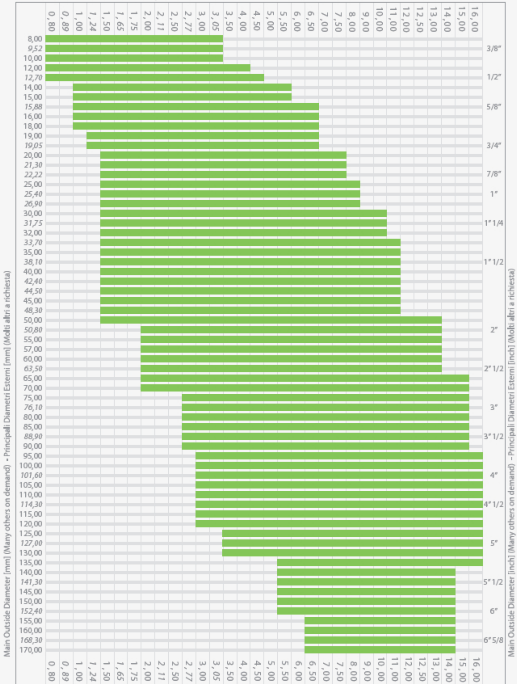
Main Wall Thickness [mm] (Many others on demand) - Principali Spessori [mm] (Molti altri a richiesta)
